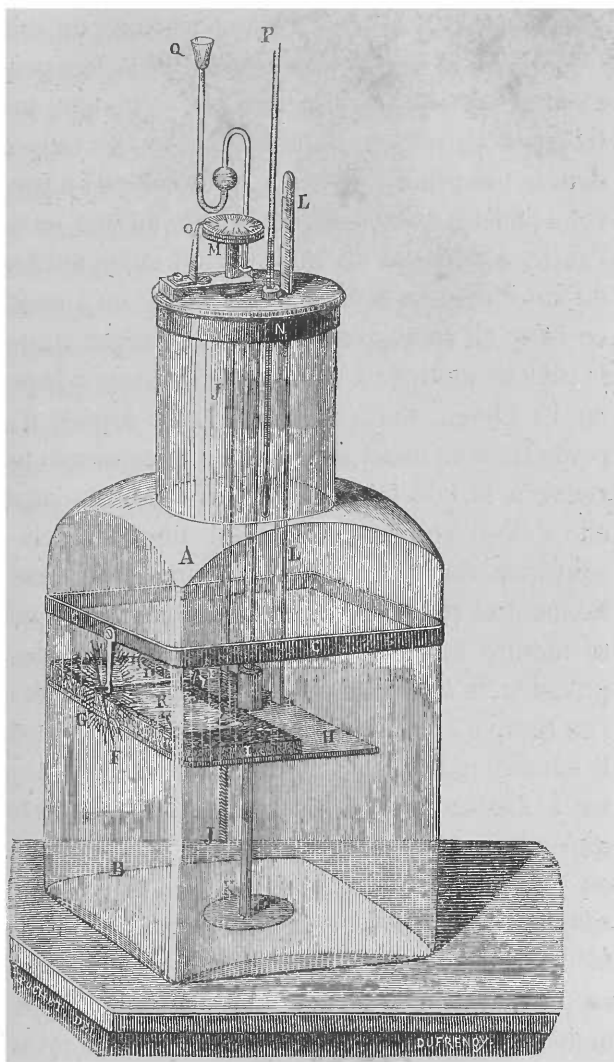
Fig. 32. — Appareil de M. Calliburcès pour mesurer les variations d'intensité des mouvements vibratiles.
