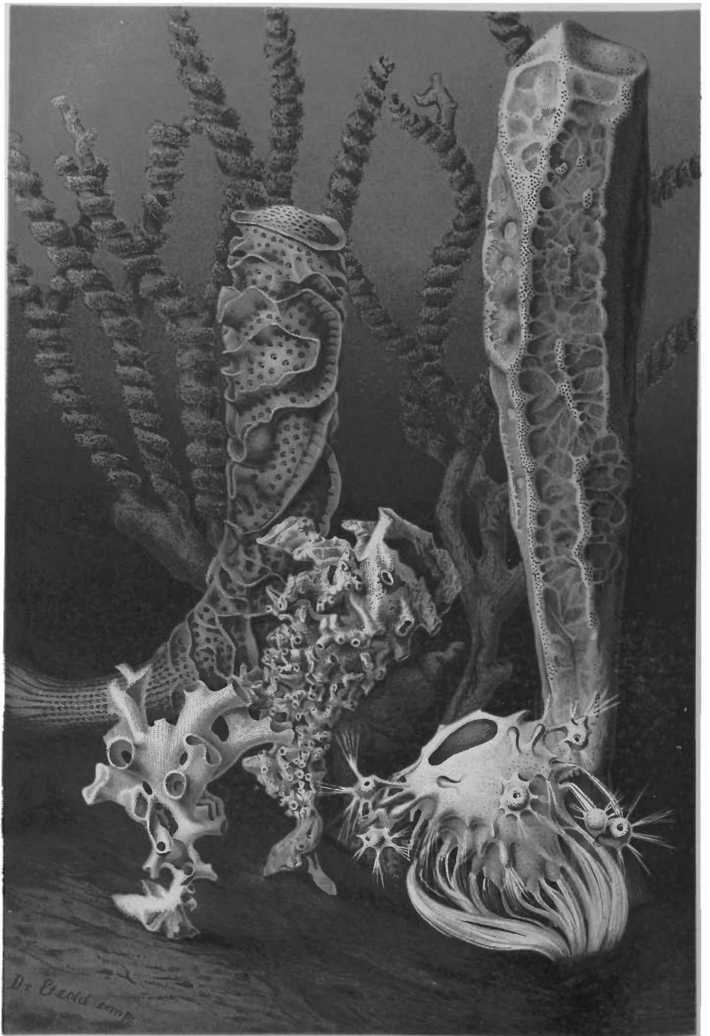
GLASSCHWÄMME (Hexactinellidae).
