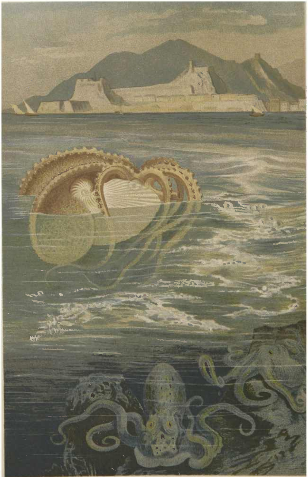
PAPIER - NAUTILUS.
