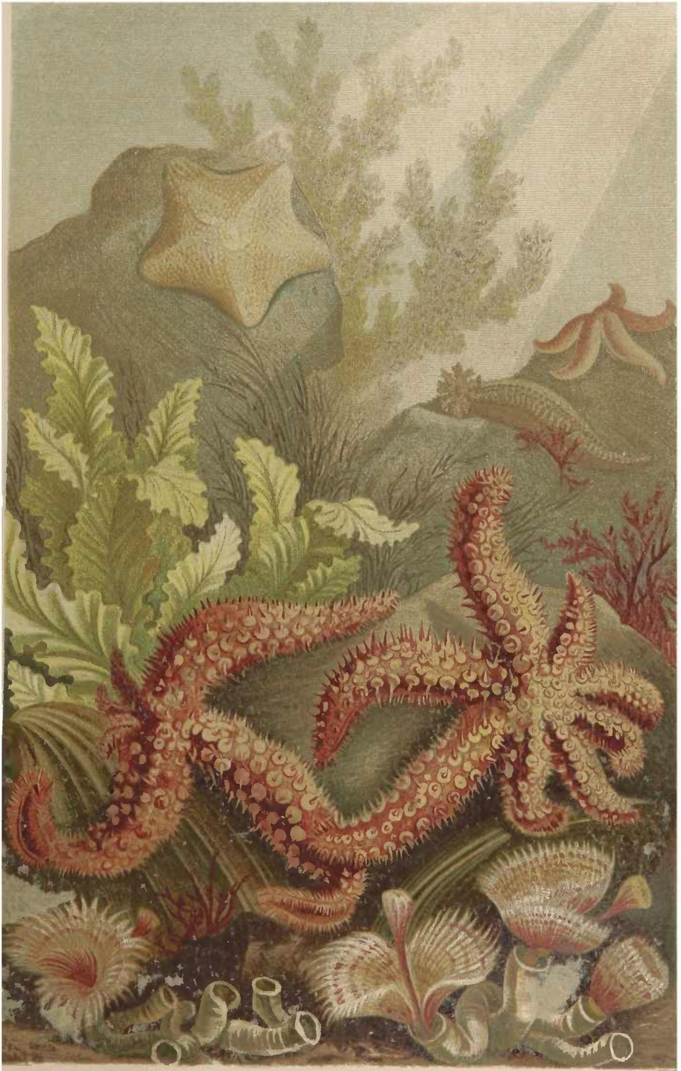
———ACHELHÄUTER.
