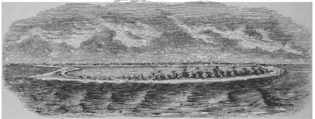
Koralleninsel oder Atoll.
