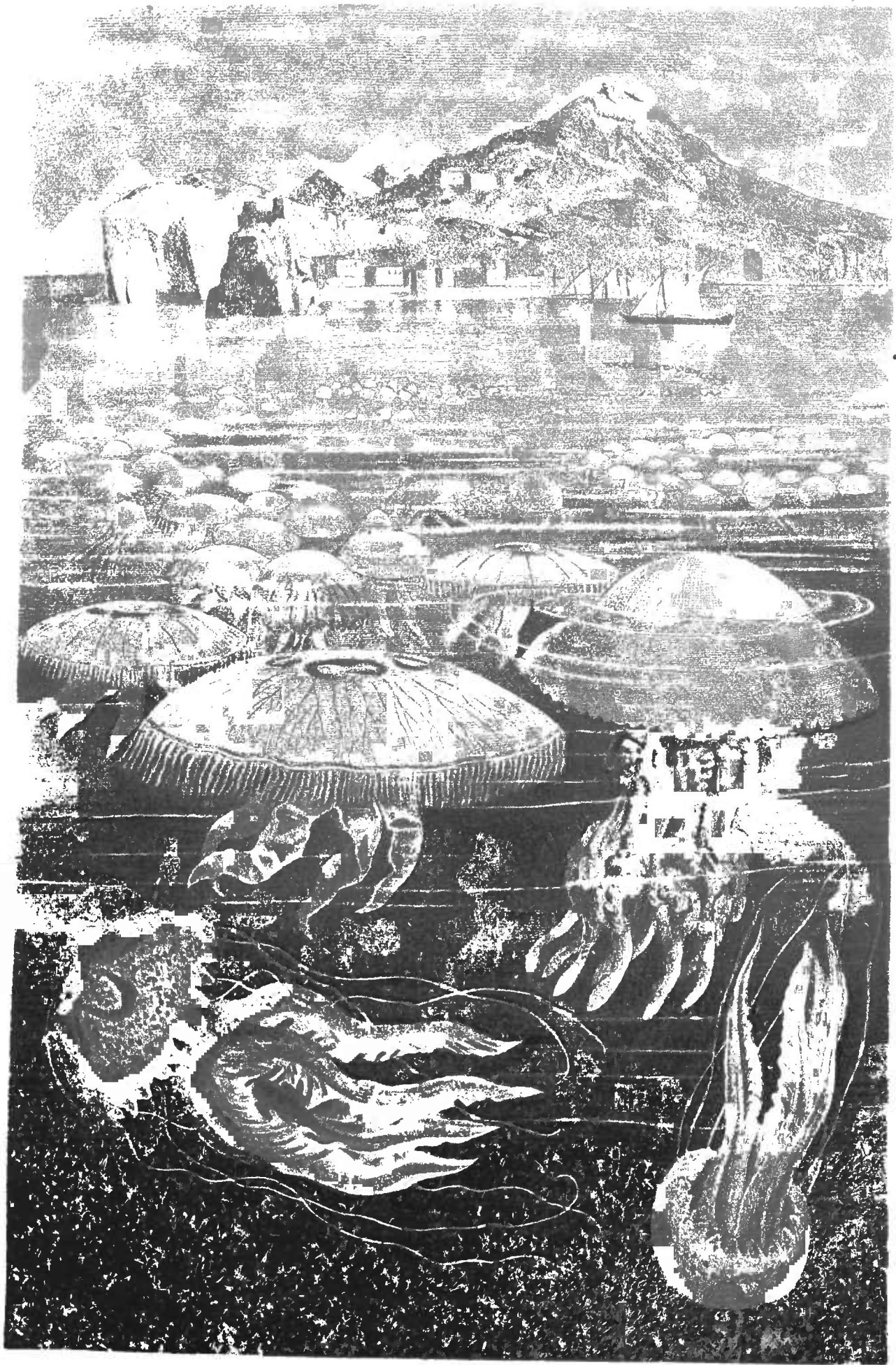
SCHIRMQUALLEN.
