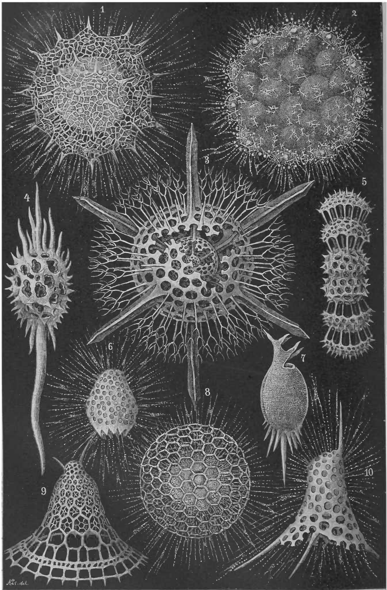
Radiolarien.
