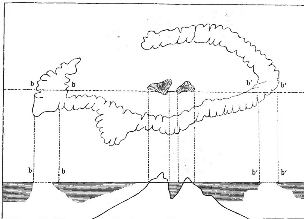
Umriss der Insel Uiva, mit projiziertem Durchschnitt.
