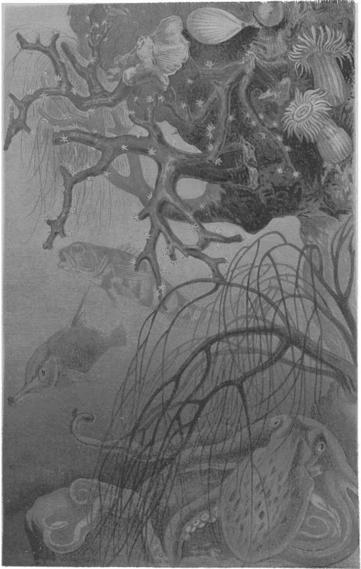
EDELKORALLE.
