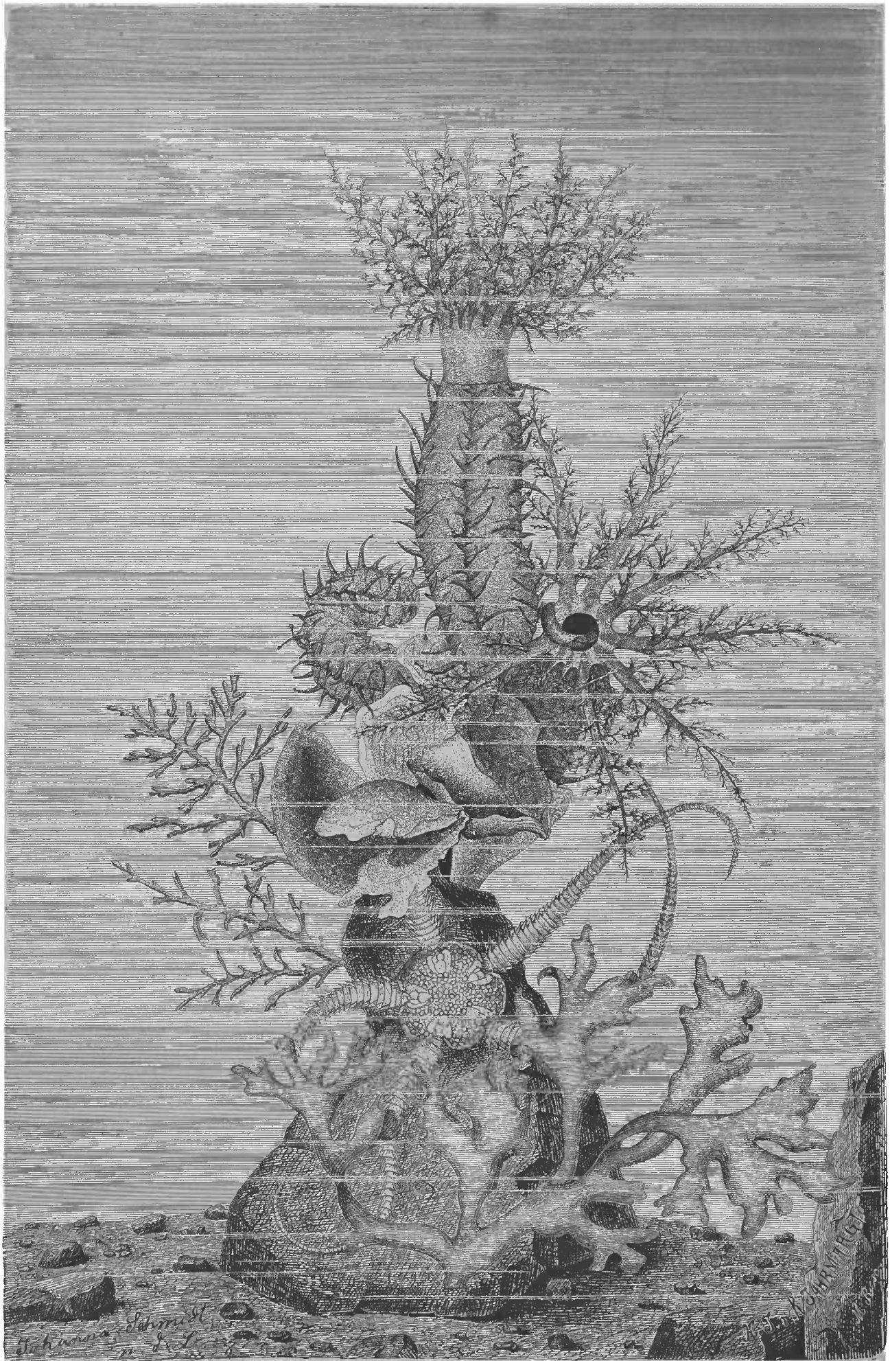
Kletterholothurie.
