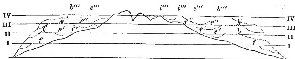
Schematischer Durchschnitt einer Insel mit Korallenriffen.
