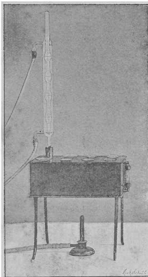
Fig. 6. — Bain-marie.
