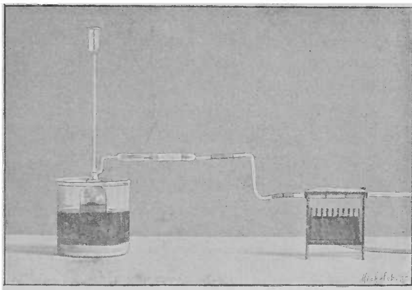
Fig. 5. — Appareil de Marsh.
