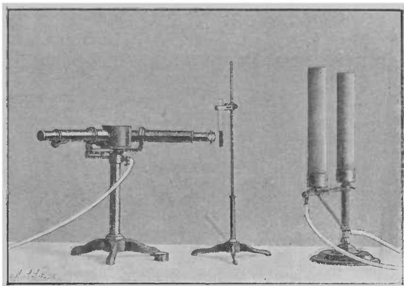
Fig. 1. — Examen spectroscopique du sang.
