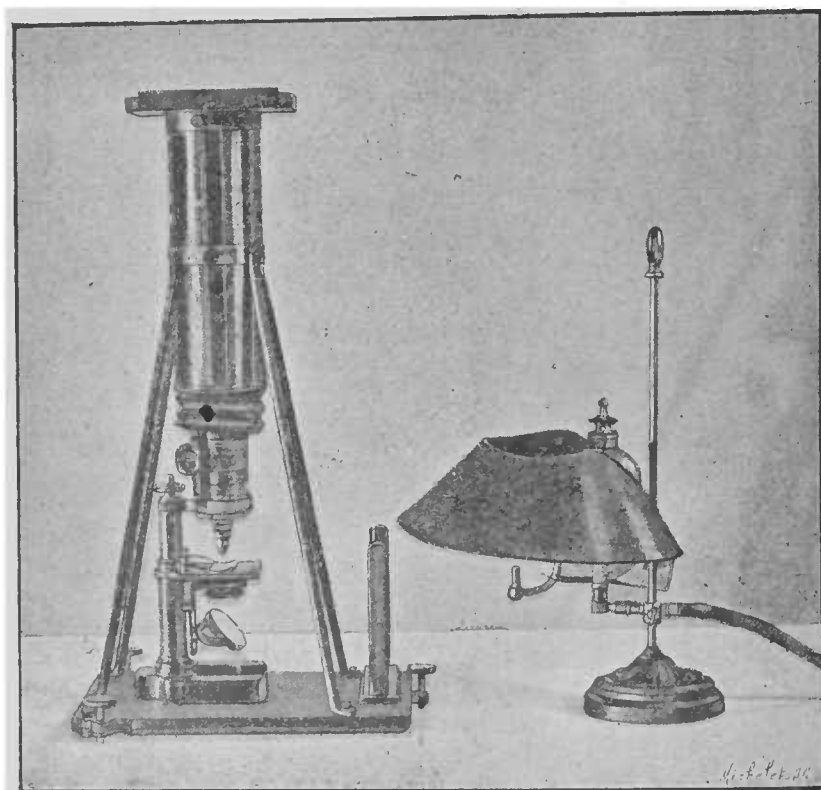
Fig. 9. — Appareil pour la photographie microscopique.
