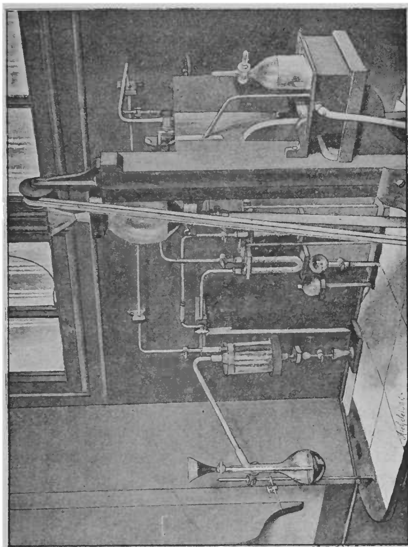
Fig. 3. — Extraction des gaz du sang.
