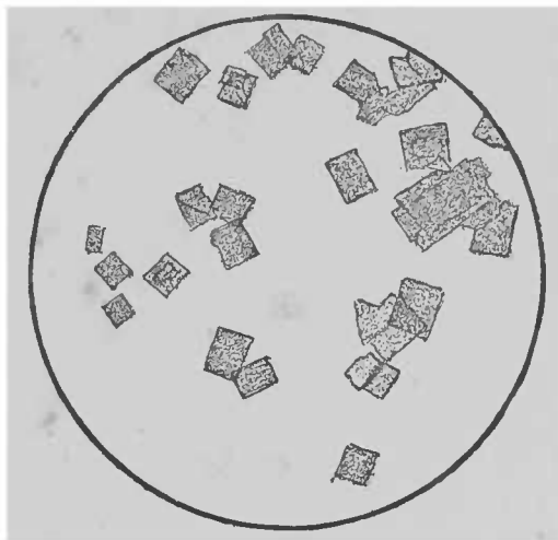
Fig. 14. — Picrate d'Atropine.
