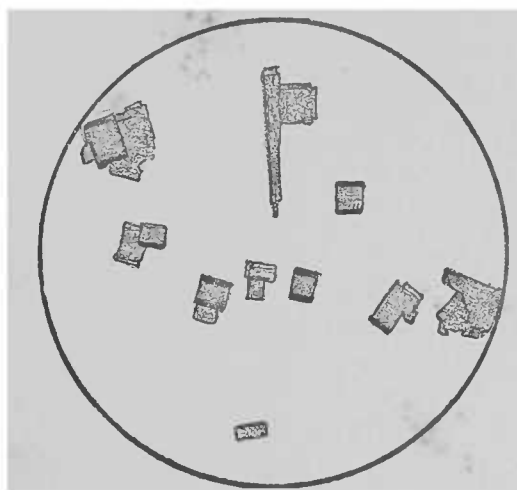
Fig. 21. — Picrate d'Hyosциamine.
