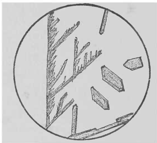
Fig 23. — Acide Picrique.
