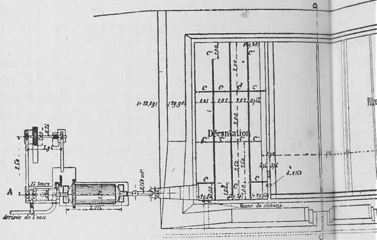
Fig. 4. — Epuration de l'eau par le système Anderson à l'usage
