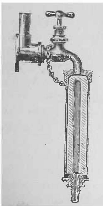
Fig. 27. — Filtre Berkefeld, filtrant de dehors en dedans.
