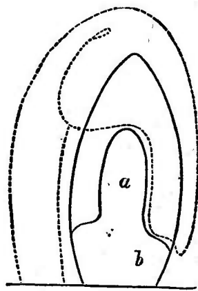
FIG. 103. — Schéma représentant la disposition d'une jeune feuille.
